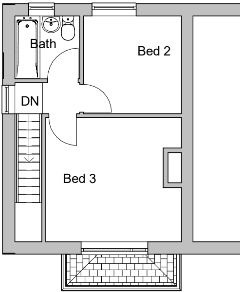
03a FF Existing 1 : 100
