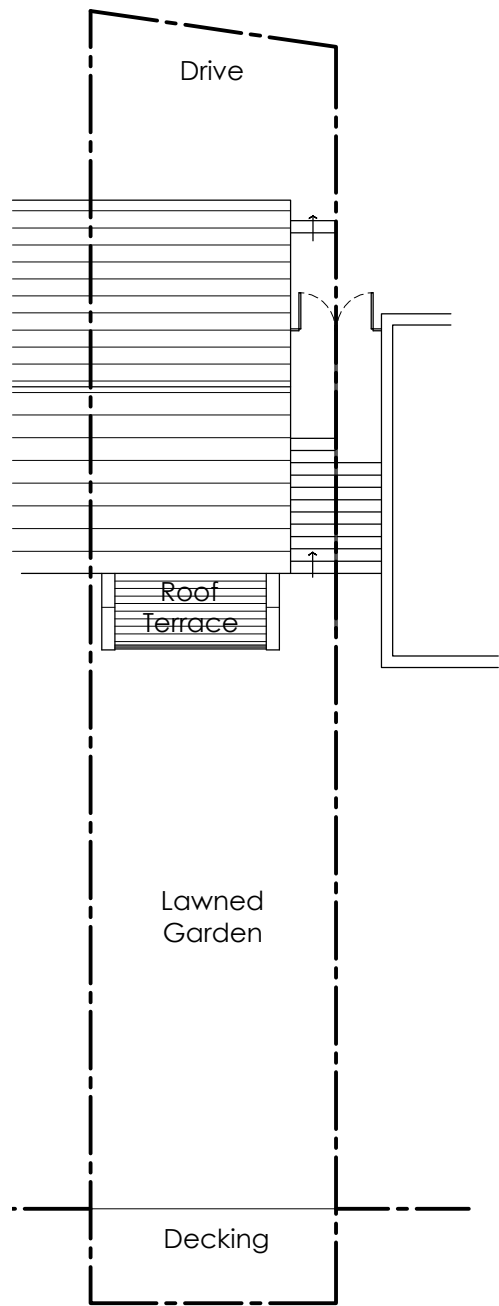
Site Plan 1:200
