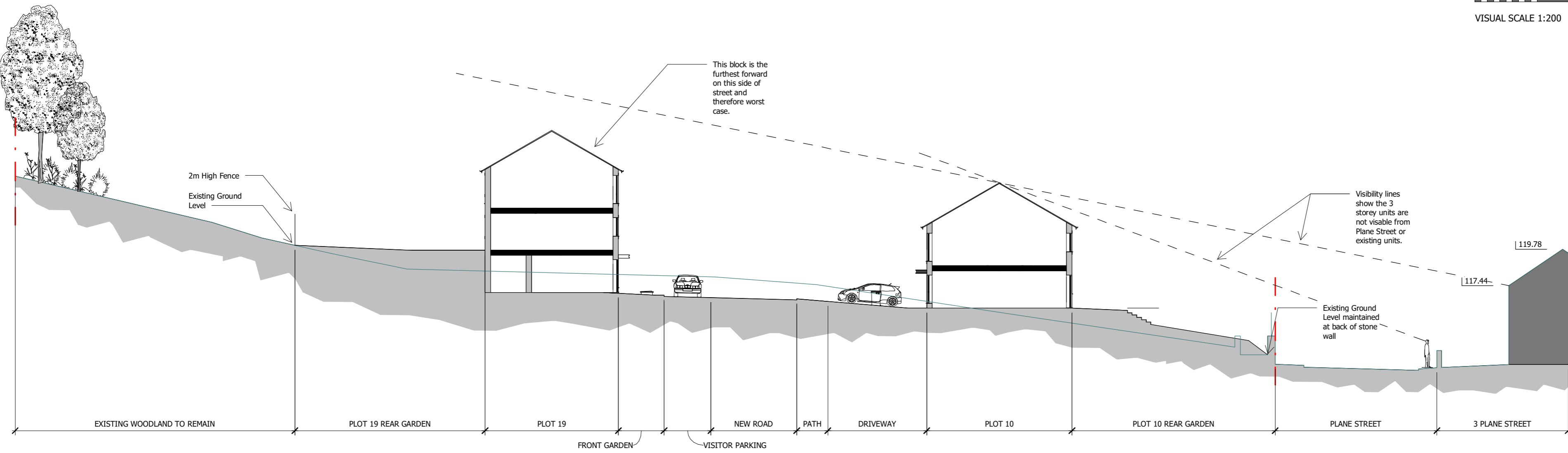
Site Section A 1 : 200
