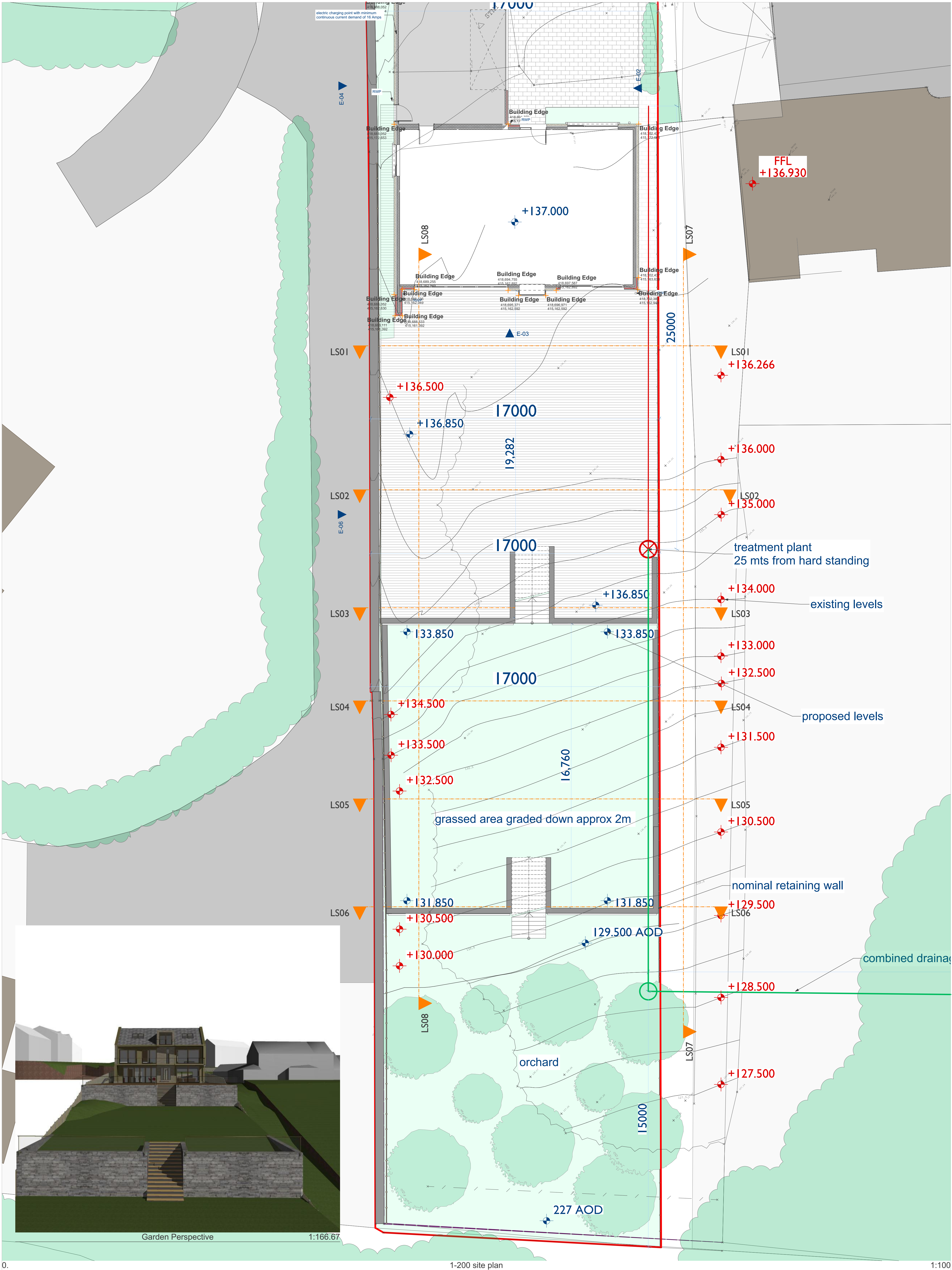
0. 1-200 site plan 1:100
