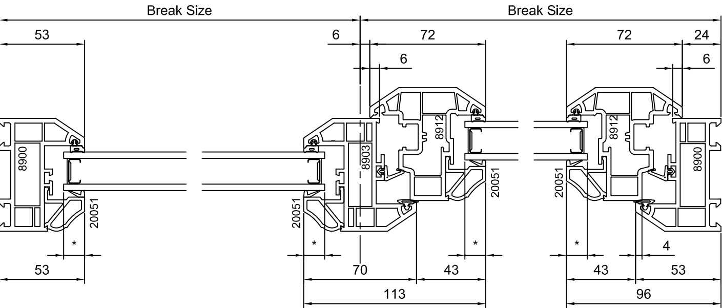
Section D-D
