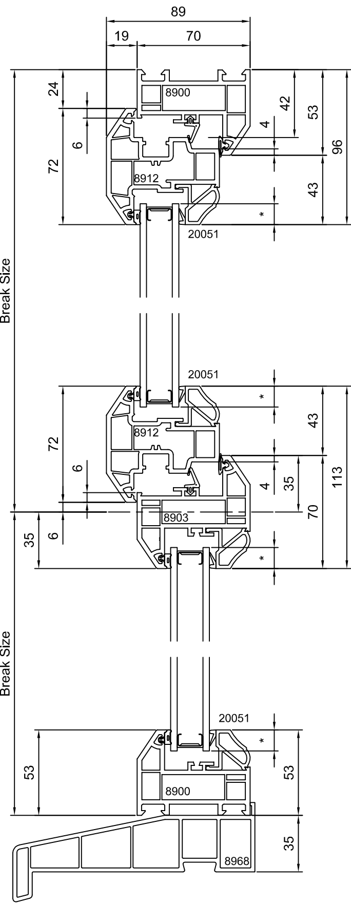
Section A-A
