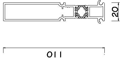
006.1970 20mm Coupler
