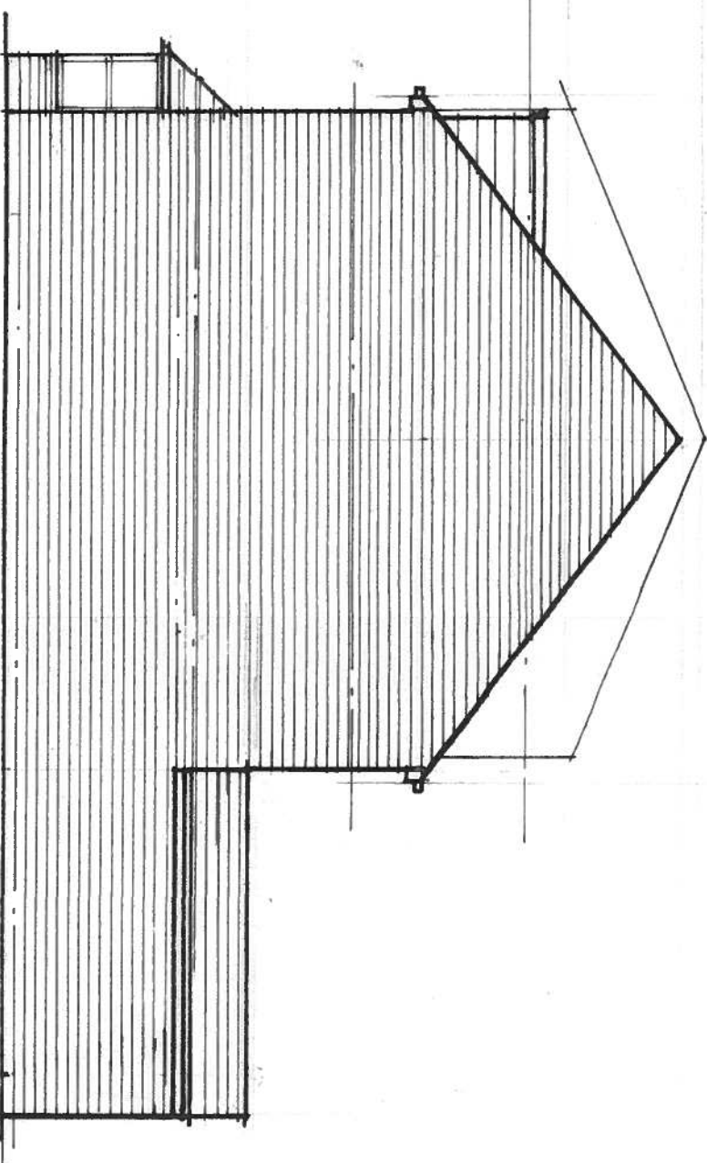
SIDE 1:100
